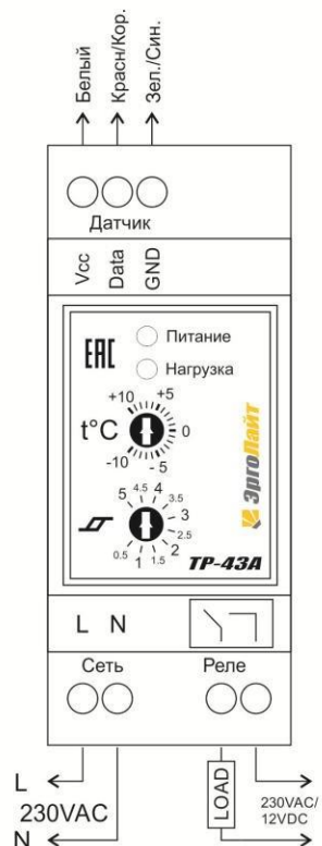
Схема 2. Подключение терморегулятора и нагрузки к разным сетям питания
