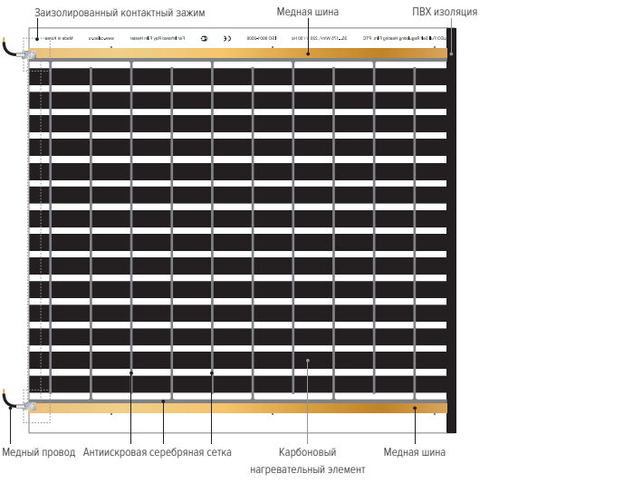
Рис. Общий вид термопленки CALEO, расположение основных ее элементов, контактных зажимов и мест подключения и изоляции
