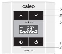
Рис. 2. Модели 330S/540S
