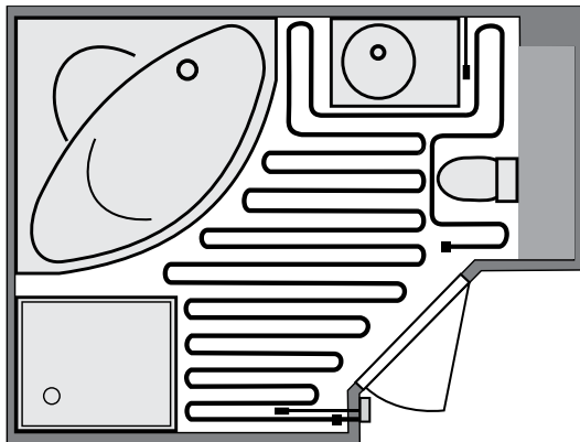
Рисунок 2 Схема укладки нагревательного кабеля
