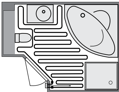
Рис. 2. Схема укладки нагревательного кабеля
