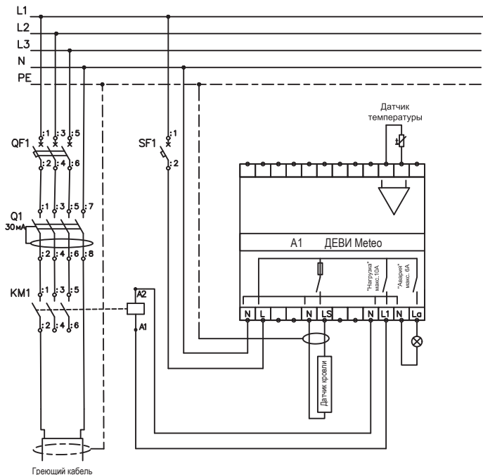
Рис. 15. Схема подключения греющего контура через контактор
