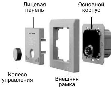
Рис. 3. Устройство терморегулятора
