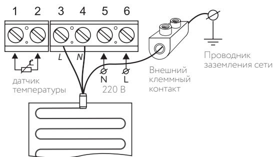
Рисунок 2. Схема подключения мата к сети (220 В)
