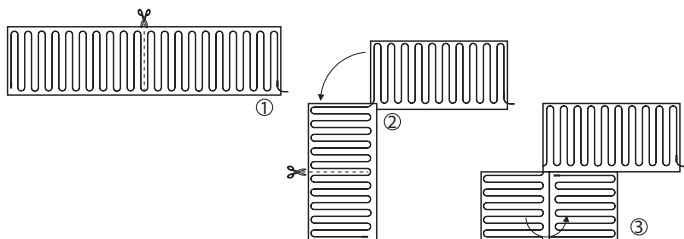
Рисунок 4. 1. Разрез мата. 2. Разворот на 90°. 3. Разворот на 180°.
